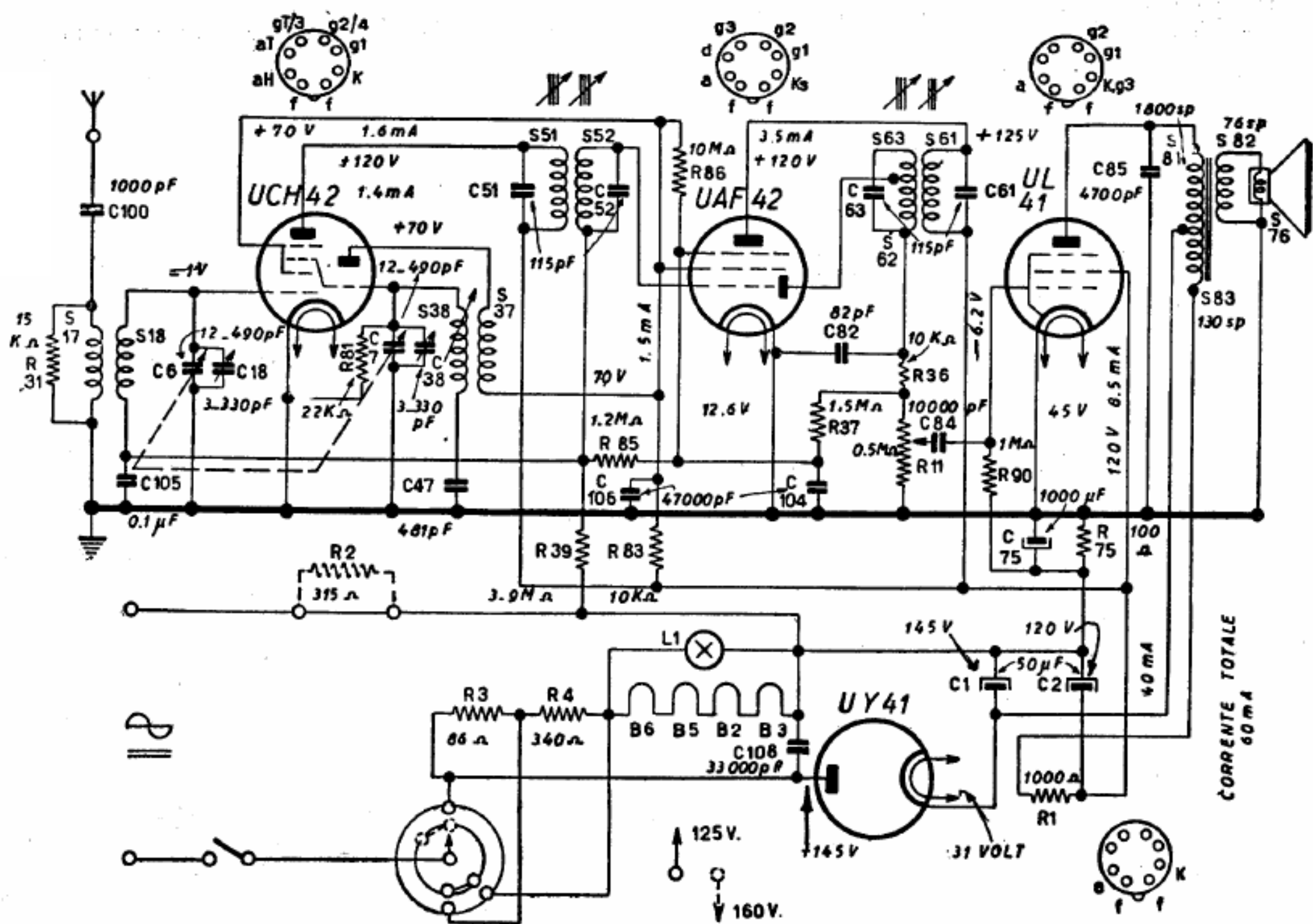
PHILIPS RADIO - Mod. BI. 191 U - Onde medie. Media frequenza 456 kc. Placca finale 125 V e 40 mA, schermo 120 V, e 8,5 mA, griglia -6,2 V.
